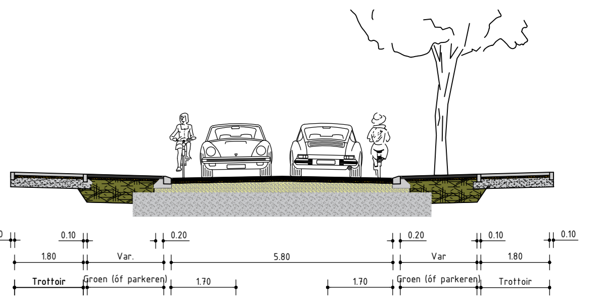
Profiel A Bergstraat SCHAAL 1 : 100
