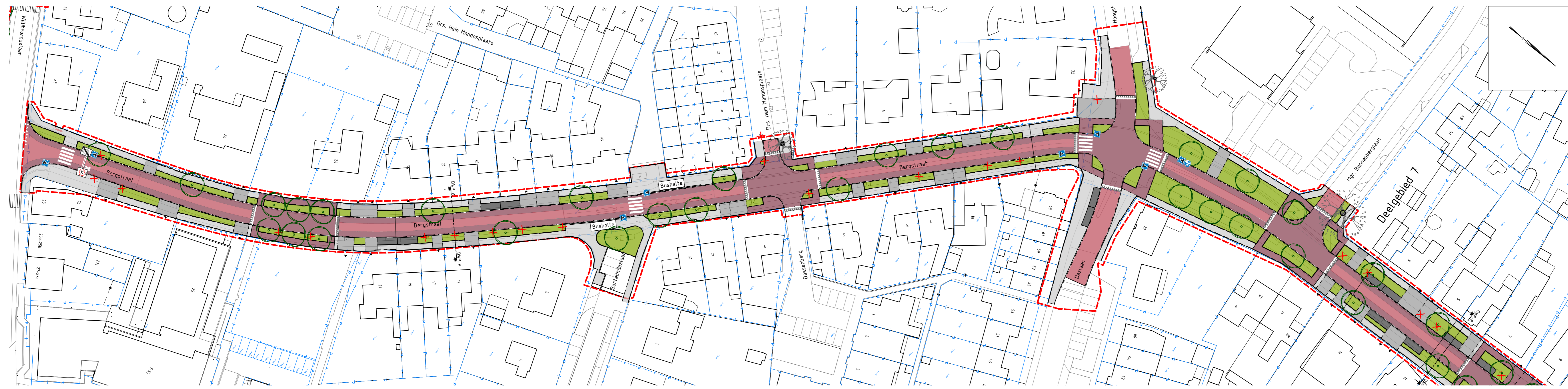
Deelgebied 6 Bergstraat Schaal 1 : 500
