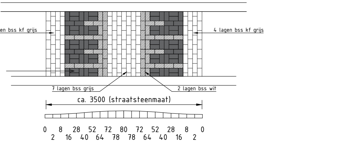
Principe detail drempel 8cm 30 km/h Schaal: 1:50
