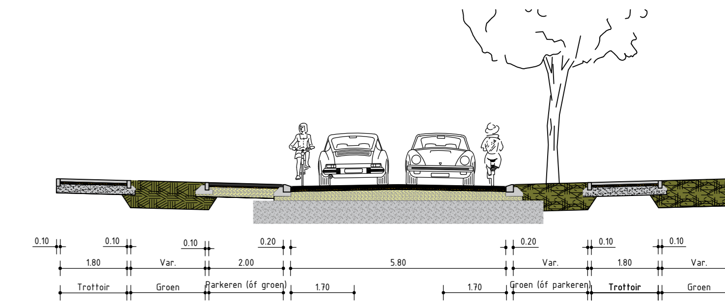
Profiel B OLV-dijk SCHAAL 1 : 100
